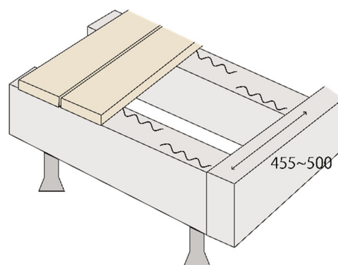
根太ピッチ 455～500mm
