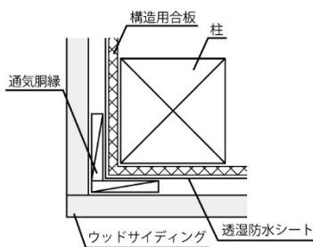
出隅 片方勝ち
