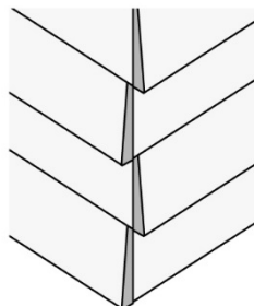
出隅 片方勝ちを横から見た図
