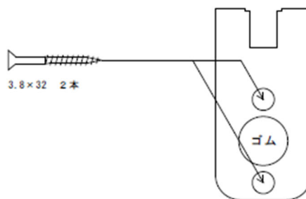
戸尻ガイド
