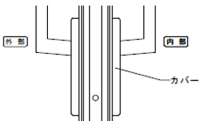
戸先立面図
