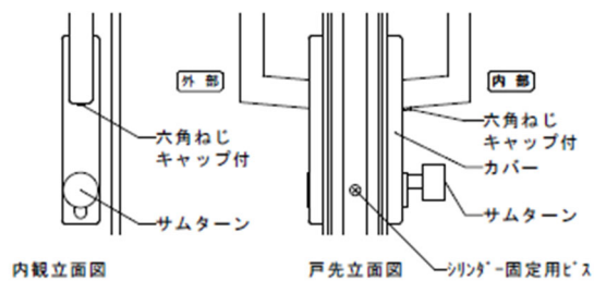
内観立面図
