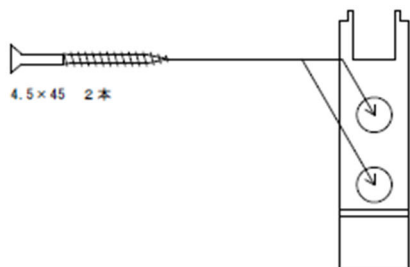
戸先ガイド
