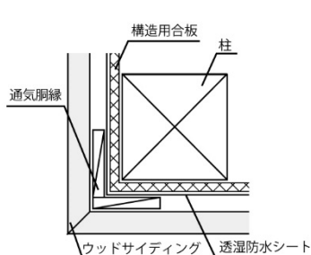
出隅 留め加工
