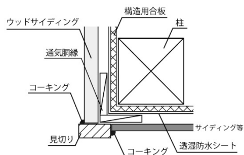
他の仕上材との切替
