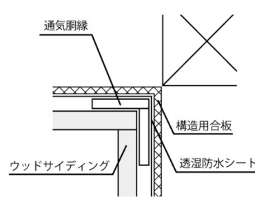
入隅 片方勝ち
