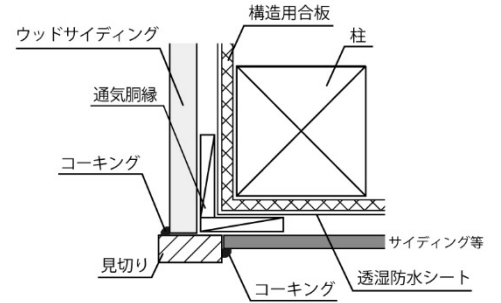
他の仕上材との切替
